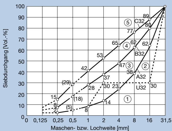
Nach Bild L.3, DIN 1045-2: Sieblinien mit einem Größtkorn von 32 mm
