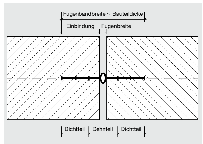
Bild 2: Einbauprinzip von innenliegenden Bewegungsfugenbändern
