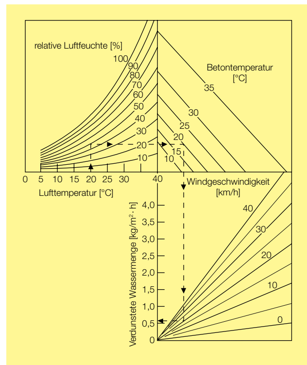
Bild 1: Das Austrocknungsverhalten von nicht geschalten Betonoberflächen in Abhängigkeit von Windgeschwindigkeit, Luftfeuchte und Temperatureinfluss [4]
