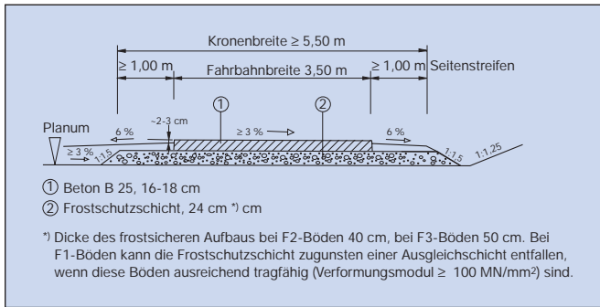
Bild 2: Regelquerschnitt eines einstreifigen Verbindungsweges mit Betondecke (größere Verkehrsbeanspruchung)
