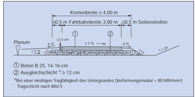
Bild 3: Regelquerschnitt eines Wirtschaftsweges mit Betondecke
