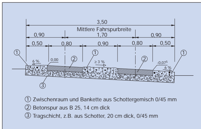
Bild 12: Regelquerschnitt eines Spurweges mit Betonspuren
