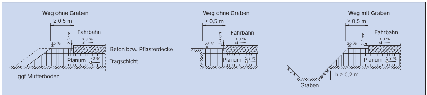
Bild 4: Randausbildung bei Betondecken mit unterschiedlicher seitlicher Ausbildung der unteren Tragschicht (nach RLW)
